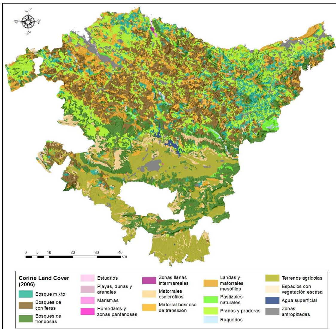
Landaretza eta lurzoruen erabilerak (Iturria: Corine Land Cover, Goeuskadin)
