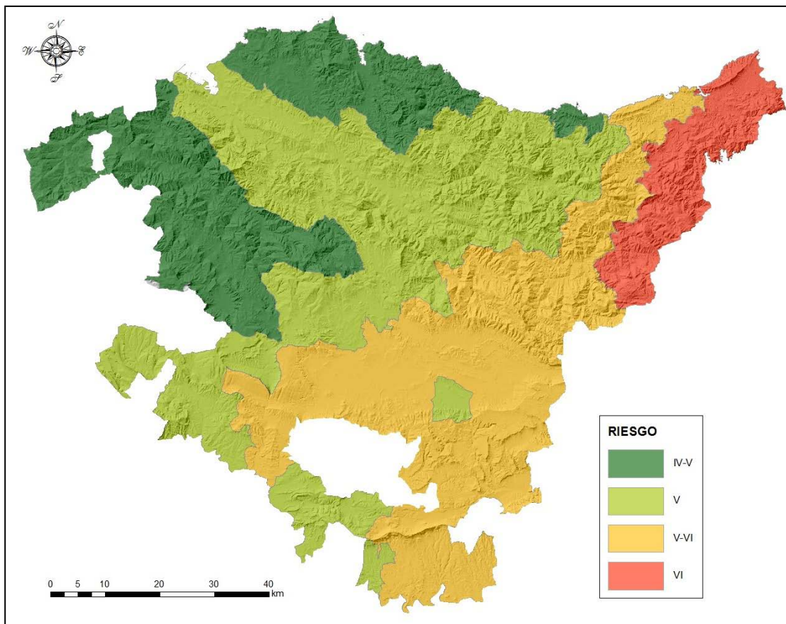
Azken intentsitate sismikoa EAerako modelizatua (Iturria: Geoeuskadi)
